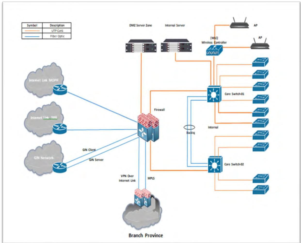
ภาพที่ ๑ ระบบเครือข่ายของกรมสนับสนุนบริการสุขภาพ
